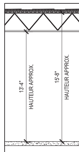
02 COUPE 01 TYPIQUE 3/16"=1'-0"
