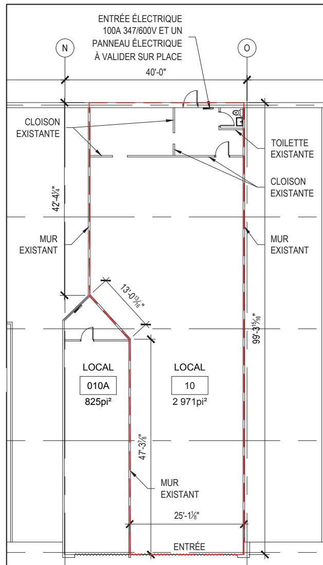
01 PLAN 01 1/16"=1'-0"
