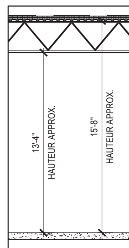
02 COUPE 01 TYPIQUE 3/16"=1'-0"
