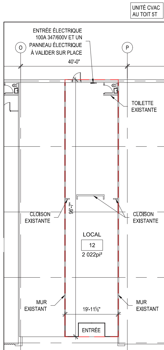
01 PLAN 01 1/16"=1'-0"
