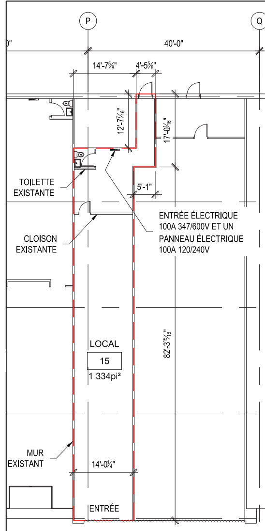
01 PLAN 01 1/16"=1'-0"
