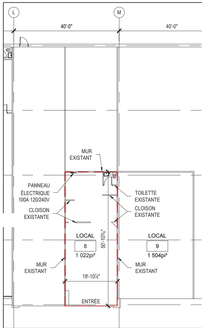
01 PLAN 1/16"=1'-0"
